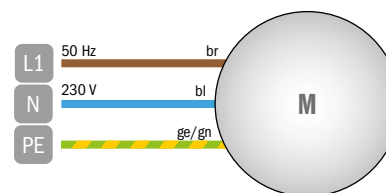
ANSCHLUSSBILD
